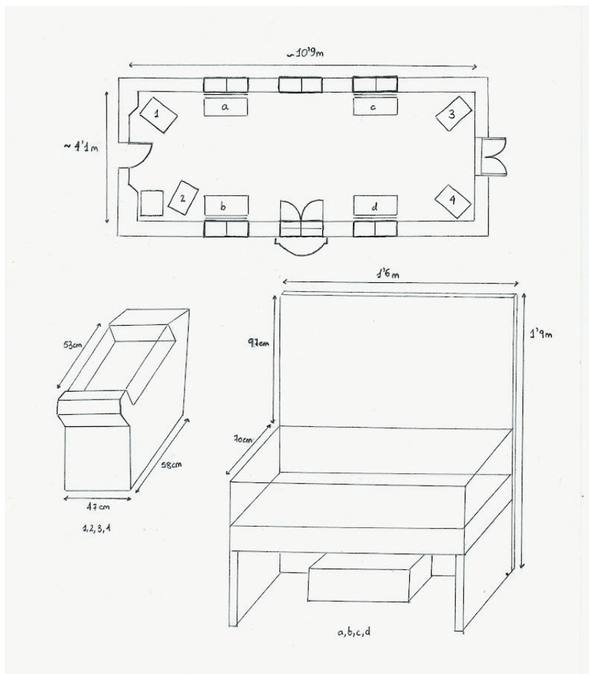
Figura 3. Plano de la sala y del equipamiento. Dibujo de Alejandro P. Elvira.
