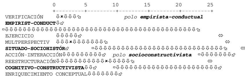
Figura 3. Conglomerados relativos a las concepciones del aprendizaje de los profesores (distancias reescaladas de 0 a 25 por la similitud de las respuestas)
