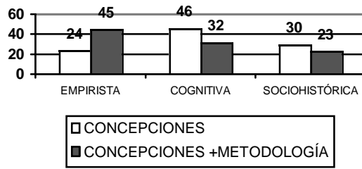
Figura 2. Valores relativos de las concepciones
