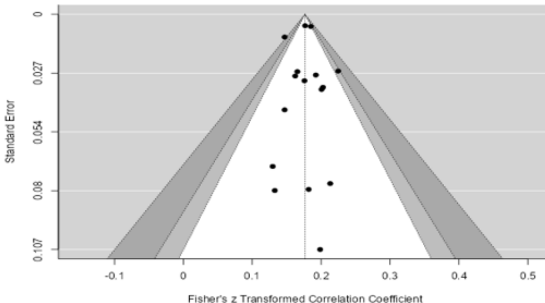
Figura 3. Funnel Plot, gráfico de dispersión.
