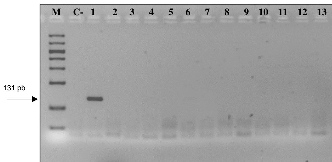
FIGURA 4. Análisis electroforético de los productos de PCR del marcador genético Alt a 1 obtenidos con los cebadores ARADIR2ALTA1/ ASOLINVALTA1 (específicos del grupo de Alternaria radicina ). Amplificación a partir de Alternaria radicina (1), A. alternata CBS 154.31(2), A. alternata CBS 117130 (3), A. alternata CBS 117143 (4), A. tenuissima (5), A. longipes (6), A. arborescens (7), A. citri (8), A. gaisen (9), A. solani (10), A. dauci (11), A. porri (12), A. infectoria (13). (C-) Control negativo sin ADN, (M) Marcador de tamaño molecular Biomarker® Low.
