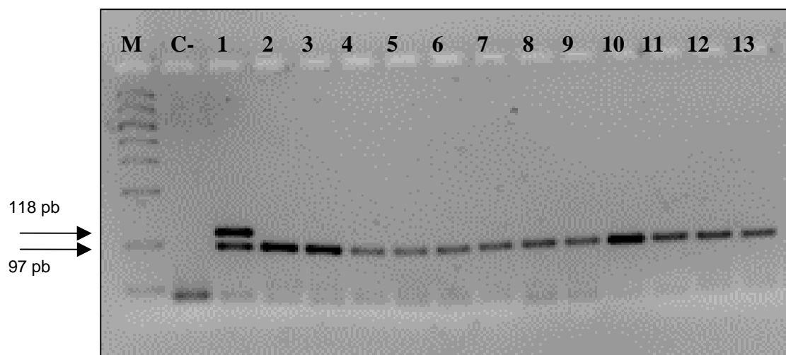
FIGURA 5. Análisis electroforético de los productos de PCR del marcador genético Alt a 1 obtenidos con los cebadores Dir3Alta1 (común del género Alternaria ) y AINFDIRALTA1/ AINFINVALTA1 (específicos del grupo de Alternaria infectoria ). Amplificación a partir de Alternaria infectoria (1), A. alternata CBS 154.31(2), A. alternata CBS 117130 (3), A. alternata CBS 117143 (4), A. tenuissima (5), A. longipes (6), A. arborescens (7), A. citri (8), A. gaisen (9), A. solani (10), A. dauci (11), A. porri (12), A. radicina (13),. (C-) Control negativo sin ADN, (M) Marcador de tamaño molecular Biomarker® Low.
