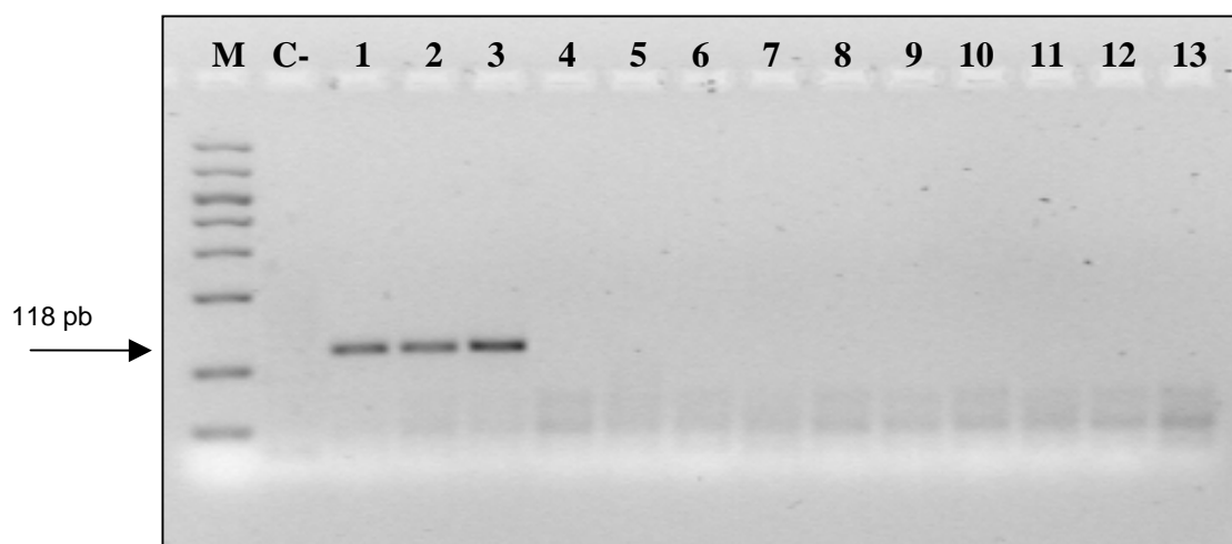
FIGURA 3. Análisis electroforético de los productos de PCR del marcador genético Alt a 1 obtenidos con los cebadores ASOLDIRALTA1/ ASOLINVALTA1 (específicos del grupo de Alternaria porri ). Amplificación a partir de Alternaria solani (1), A. dauci (2), A. porri (3), A. alternata CBS 154.31(4), A. alternata CBS 117130 (5), A. alternata CBS 117143 (6), A. tenuissima (7), A. longipes (8), A. arborescens (9), A. citri (10), A. gaisen (11), A. infectoria (12), A. radicina (13). (C-) Control negativo sin ADN, (M) Marcador de tamaño molecular Biomarker® Low.
