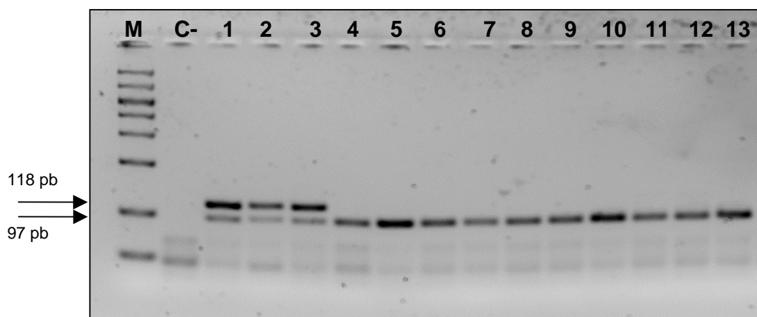
FIGURA 6. Análisis electroforético de los productos de PCR del marcador genético Alt a 1 obtenidos con los cebadores Dir3Alta1 (común del género Alternaria ) y ASOLDIRALTA1/ ASOLINVALTA1 (específicos del grupo de Alternaria porri ). Amplificación a partir de Alternaria solani (1), A. dauci (2), A. porri (3), A. alternata CBS 154.31(4), A. alternata CBS 117130 (5), A. alternata CBS 117143 (6), A. tenuissima (7), A. longipes (8), A. arborescens (9), A. citri (10), A. gaisen (11), A. infectoria (12), A. radicina (13). (C-) Control negativo sin ADN, (M) Marcador de tamaño molecular Biomarker® Low.
