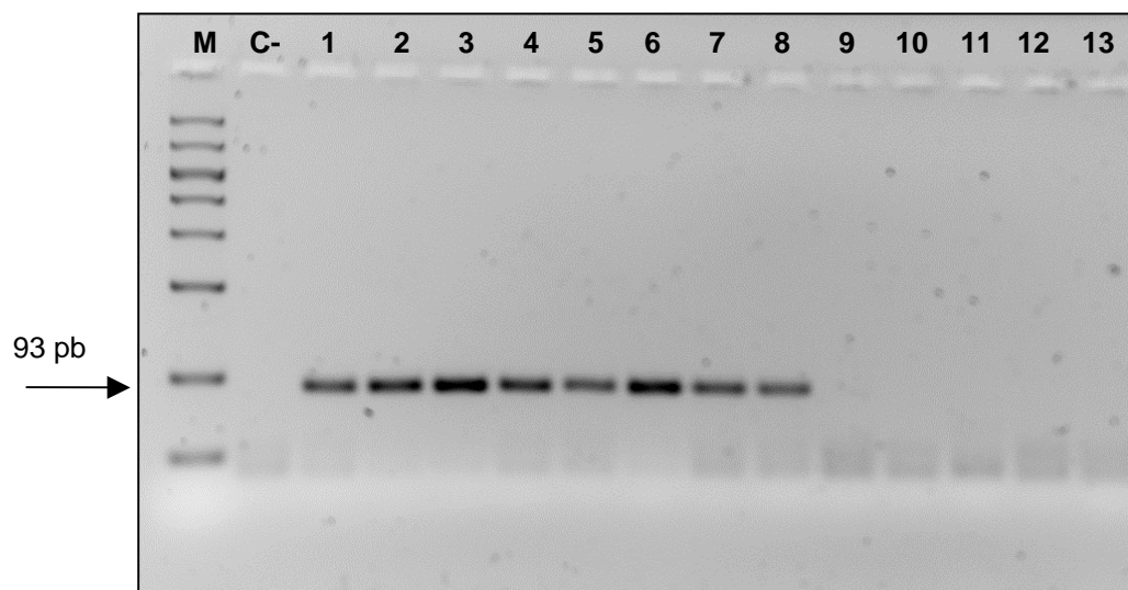
FIGURA 1. Análisis electroforético de los productos de PCR del marcador genético Alt a 1 obtenidos con los cebadores AALTDIRALTA1/ AALTINV2ALTA1 (específicos del grupo de Alternaria alternata ). Amplificación a partir de A. alternata CBS 154.31(1), A. alternata CBS 117130 (2), A. alternata CBS 117143 (3), A. tenuissima (4), A. longipes (5), A. arborescens (6), A. citri (7), A. gaisen (8), A. solani (9), A. dauci (10), A. porri (11), A. radicina (12), A. infectoria (13). (C-) Control negativo sin ADN, (M) Marcador de tamaño molecular Biomarker® Low.
