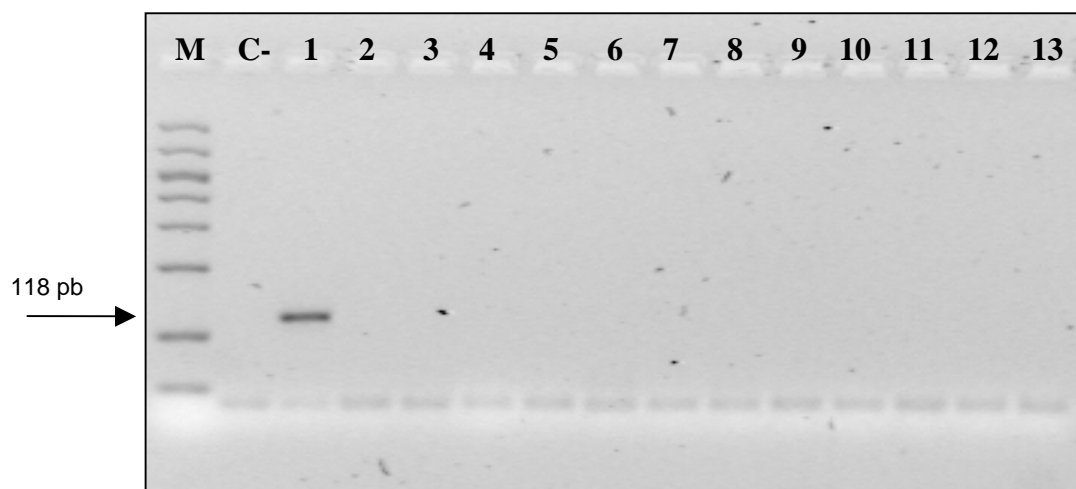
FIGURA 2. Análisis electroforético de los productos de PCR del marcador genético Alt a 1 obtenidos con los cebadores AINFDIRALTA1/ AINFINVALTA1 (específicos del grupo de Alternaria infectoria ). Amplificación a partir de Alternaria infectoria (1), A. alternata CBS 154.31(2), A. alternata CBS 117130 (3), A. alternata CBS 117143 (4), A. tenuissima (5), A. longipes (6), A. arborescens (7), A. citri (8), A. gaisen (9), A. solani (10), A. dauci (11), A. porri (12), A. radicina (13),. (C-) Control negativo sin ADN, (M) Marcador de tamaño molecular Biomarker® Low.
