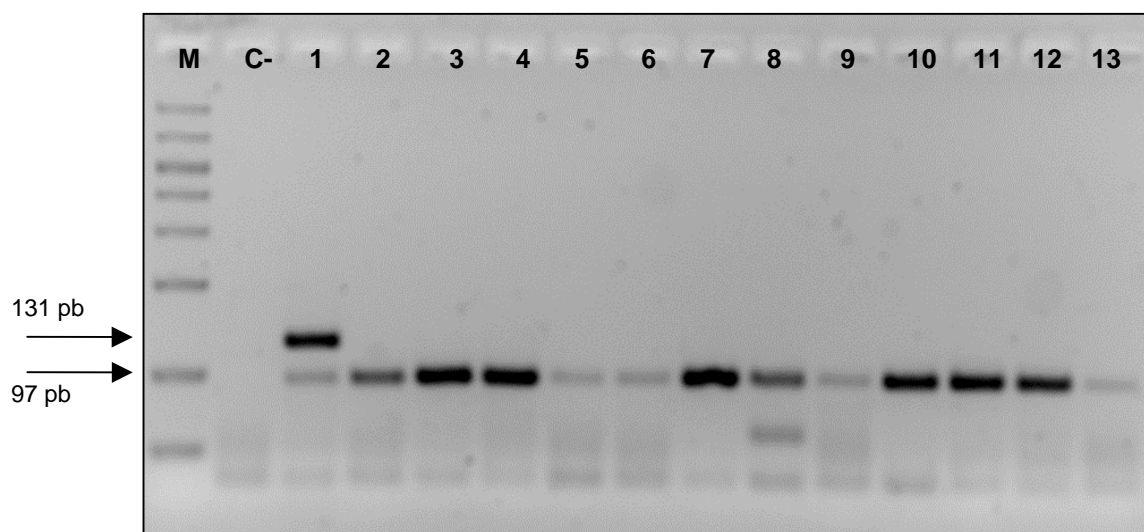
FIGURA 7. Análisis electroforético de los productos de PCR del marcador genético Alt a 1 obtenidos con los cebadores Dir3Alta1 (común del género Alternaria ) y ARADIR2ALTA1/ ASOLINVALTA1 (específicos del grupo de Alternaria radicina ). Amplificación a partir de Alternaria radicina (1), A. alternata CBS 154.31(2), A. alternata CBS 117130 (3), A. alternata CBS 117143 (4), A. tenuissima (5), A. longipes (6), A. arborescens (7), A. citri (8), A. gaisen (9), A. solani (10), A. dauci (11), A. porri (12), A. infectoria (13). (C-) Control negativo sin ADN, (M) Marcador de tamaño molecular Biomarker® Low.
