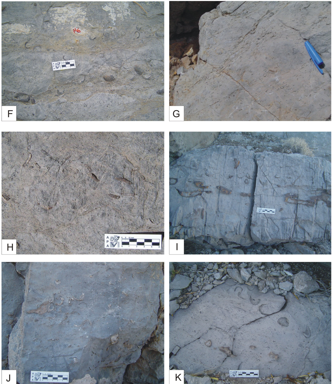
Fig. 3. (Esta página y la previa) A- Aspecto general de la Unidad 1 en la Barda 2; B- Detalle de ciclos de somerización. Observar intervalos centimétricos de packstone a grainstone de las calizas en la base (concentraciones bioclásticas de tipo B) (escala: 15 cm); C a K- Concentraciones fósiles en la Formación La Manga: C- Tipo A, concentraciones fósiles canalizadas de Gryphaea sp.; D- Tipo B, concentraciones de conchillas de Gryphaea sp. fuertemente retrabajadas; E- Tipo C, concentraciones de conchillas de Gryphaea sp. moderadamente retrabajadas; F- Tipo D, concentraciones de Gryphaea sp. con matriz biomicrítica y biopelmicrítica; G- Tipo E, detrito de conchillas (escala: 4 cm); H- Tipo F, concentraciones de espinas de equinodermos producidas por corrientes de fondo (vista en planta); I- Tipo F, concentraciones producidas por corrientes de fondo (sección perpendicular a la estratificación) donde se observa un nivel de corales y un nivel de grifeidos; J- Tipo G, concentraciones de conchillas en agrupaciones; K- Asociaciones de concentraciones de fósiles tipo E y F.
