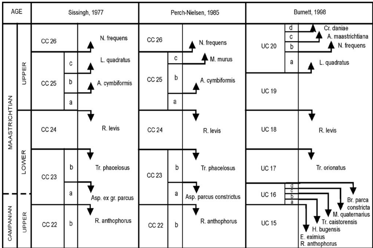
Fig. 2.- Summary of the nannofossil biozonation of Sissingh (1977), Perch-Nielsen (1985) and Burnett (1998). Fig. 2.- Resumen de las biozonaciones de Sissingh (1977), Perch-Nielsen (1985) y Burnett (1998).
