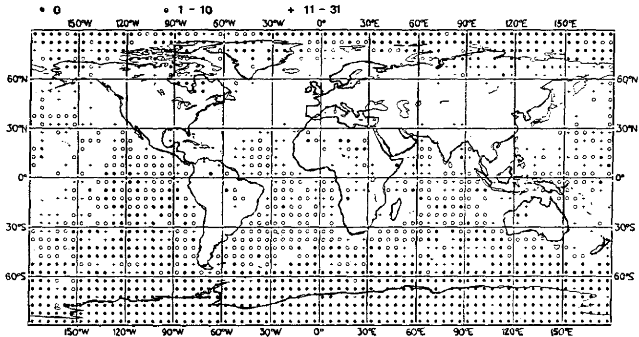
Figura 2.—Número promedio de observaciones convencionales, disponibles para el modelo de análisis a las 12Z, en el mes de julio de 1989, excluyendo datos de satélite, en cada cuadrado de 5×5 grados. Las áreas en blanco indican un mínimo de 30 observaciones. Los símbolos indican escasez de datos, como se indica en la parte superior del gráfico.
