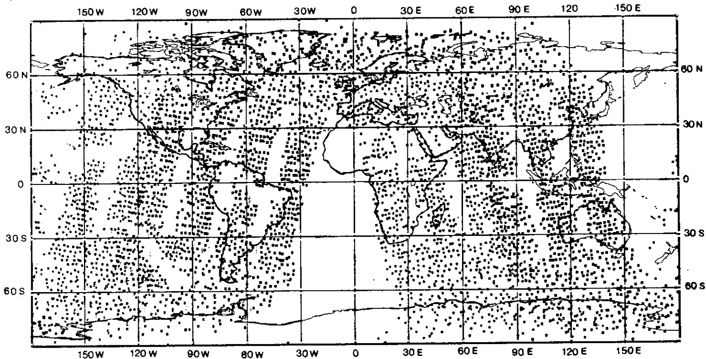
Figura 3. Cobertura de sondeos de satélites para los análisis de las 06Z y de las 12Z.
