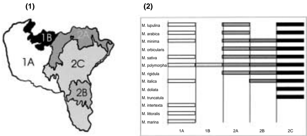
Figura 4. (1) Cartografía de los sectores y subsectores bioclimáticos para el área de trabajo (a partir de Costa et al. , 1999); (2) Representación gráfica de la caracterización bioclimática por especie: 1A= subsector miniense, 1B= subsector geresiano-queixense, 2A= subsector maragato-sanabriense, 2B= sector salmantino, 2C=sector lusitanoduriense.
