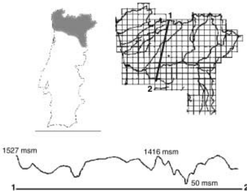
Figura 1. Localización del área de trabajo, con la representación de un perfil transversal entre la Sierra de Larouco -1- y la villa de Castro d'Aire -2-, atravesando el río Duero (50 msm).
