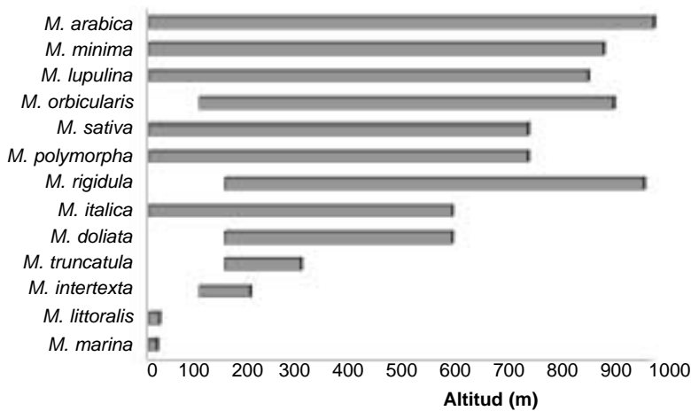
Figura 3. Representación de los intervalos altitudinales por especie para el área de trabajo.
