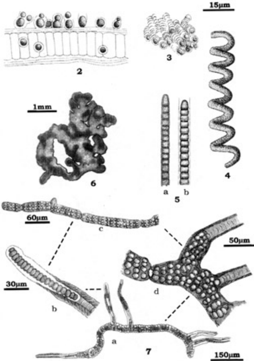
Figura 2.— Chamaesiphon minutus sobre Tolypothrix . Fig. 3, Cyanostylon sp. Fig. 4, Arthrospira skujae . Fig. 5, Symploca laete-viridis : a, tricoma desprovisto de vaina; b, filamento. Fig. 6, Rivularia hansgirgi : visión general del talo. Fig. 7, Stigonema mirabile : a, aspecto general del filamento; b, rama hormogonífera; c, inicio del desarrollo de las ramificaciones. En el tricoma se aprecia la disposición en filas de las células; d, detalle de la base de las ramas de un filamento adulto en donde se observa la estructura pluriestratificada del tricoma.
