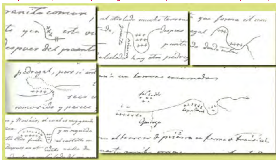
Figura 6. Ejemplos de esbozos cartográficos de las terrazas del río Sil realizados por Schulz. Su aparente simplicidad no impide una geolocalización aproximada mediante trabajo de campo.
