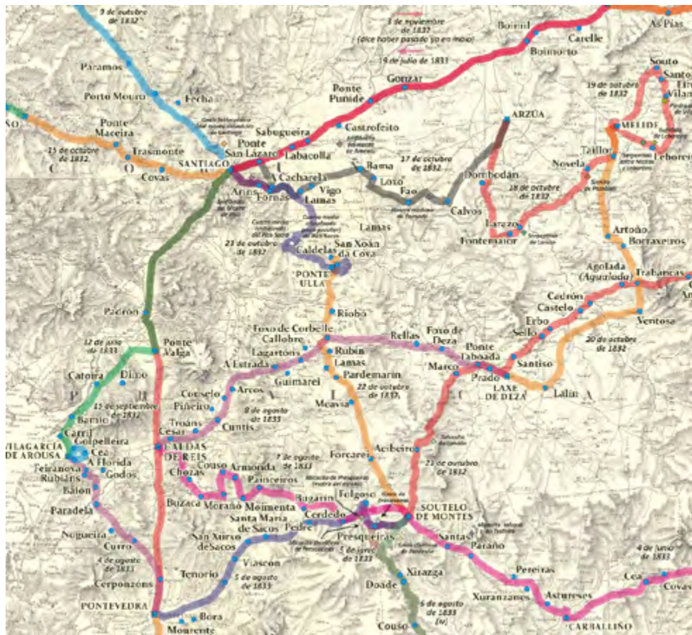
Figura 5. Transeptos geognósticos realizados por Schulz y descritos en sus cuadernos en el sector encuadrado entre las localidades de Santiago de Compostela, Melide, O Carballiño, Pontevedra y Vilagarcía de Arousa.
